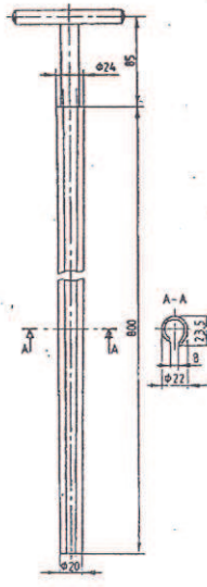
Σχήμα 5: Δειγματοληπτικό για γάλα σε άνοιξη (όλες οι διαστάσεις σημειώνονται σε mm).
