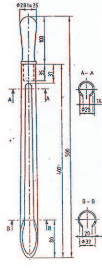
Σχήμα 6: Δειγματοληπτικό για γάλα σε άνοιξη (όλες οι διαστάσεις σημειώνονται σε mm).
